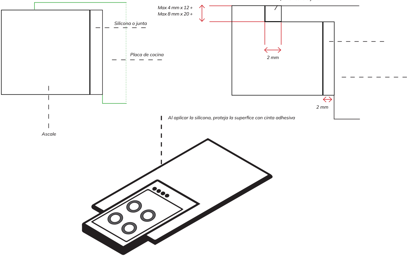
Placa de cocina sobre la encimera
